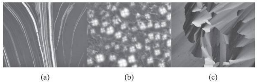
(a) ラメラ液晶 (oily streaks), (b) ラメラ液晶 (maltose cross), (c) ヘキサゴナル液晶の偏光顕微鏡観察像
